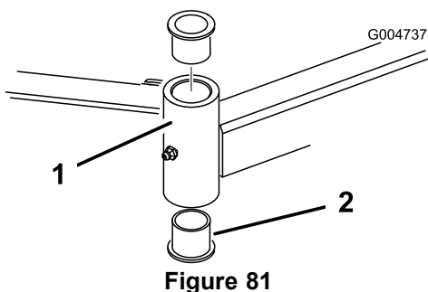
1. Tube du bras pivotant 2. Bagues
