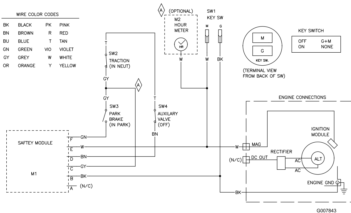
Schéma électrique — Modèle 22970 (Rev. A)
