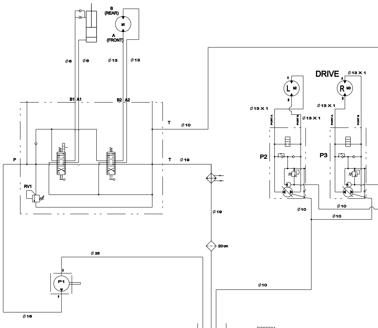
Schéma hydraulique — Modèle 22971 et 22974 (Rev. A)
