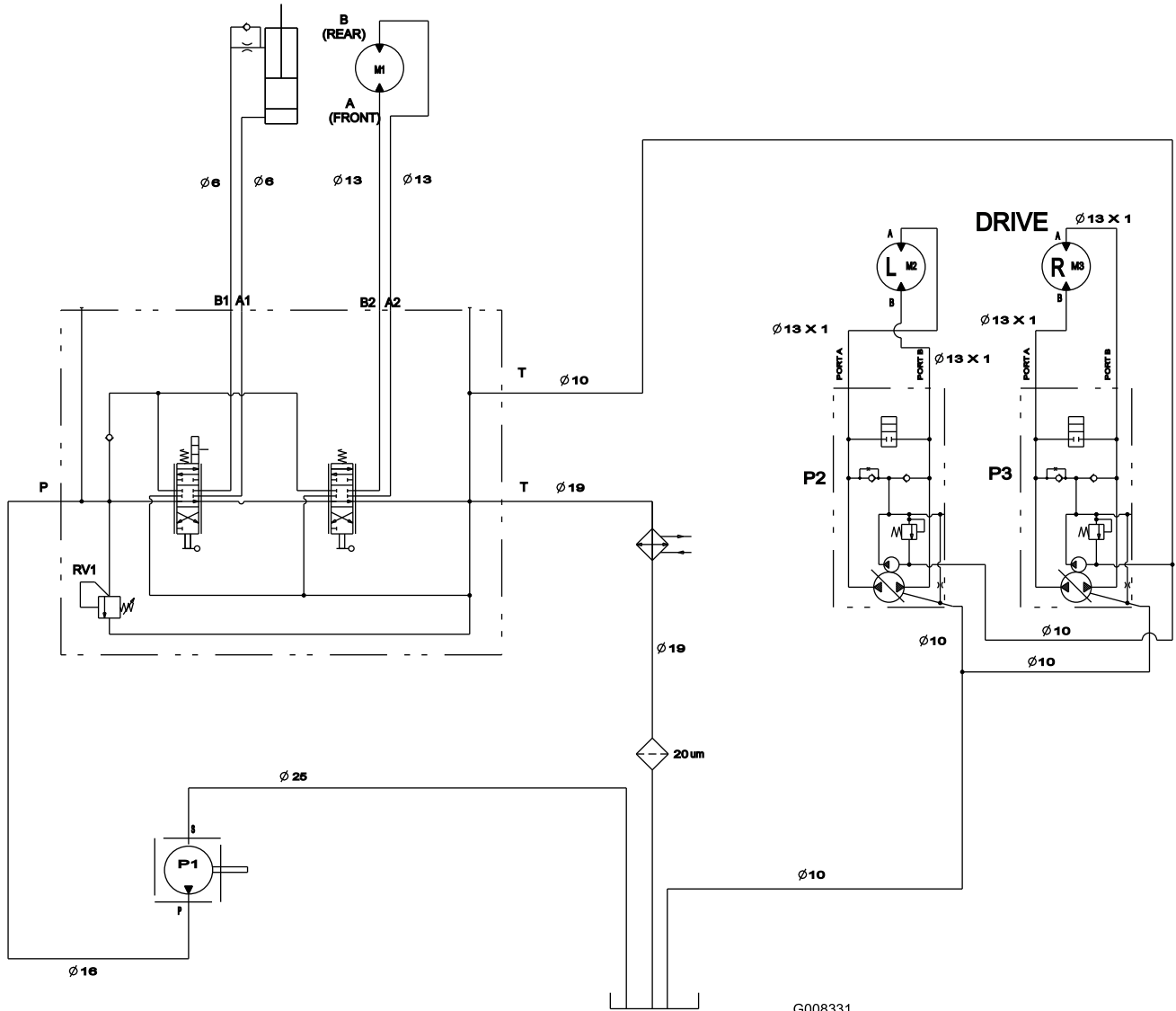
Schema Idraulico - Modello 22971e 22974 (Rev. A)
