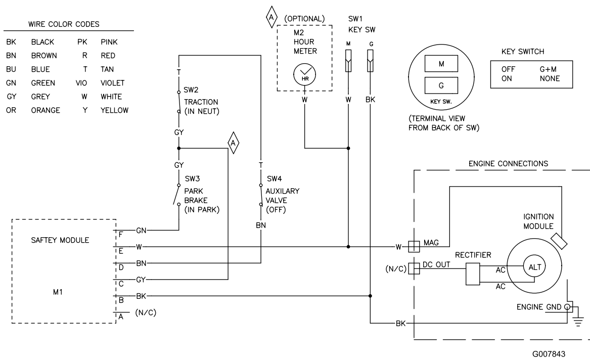
Schema Elettrico - Modello 22970 (Rev. A)
