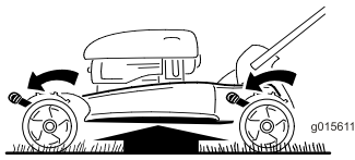
Рисунок 11 Raise the machine
