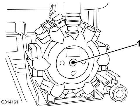
Bild 33 Pumpenmitte
