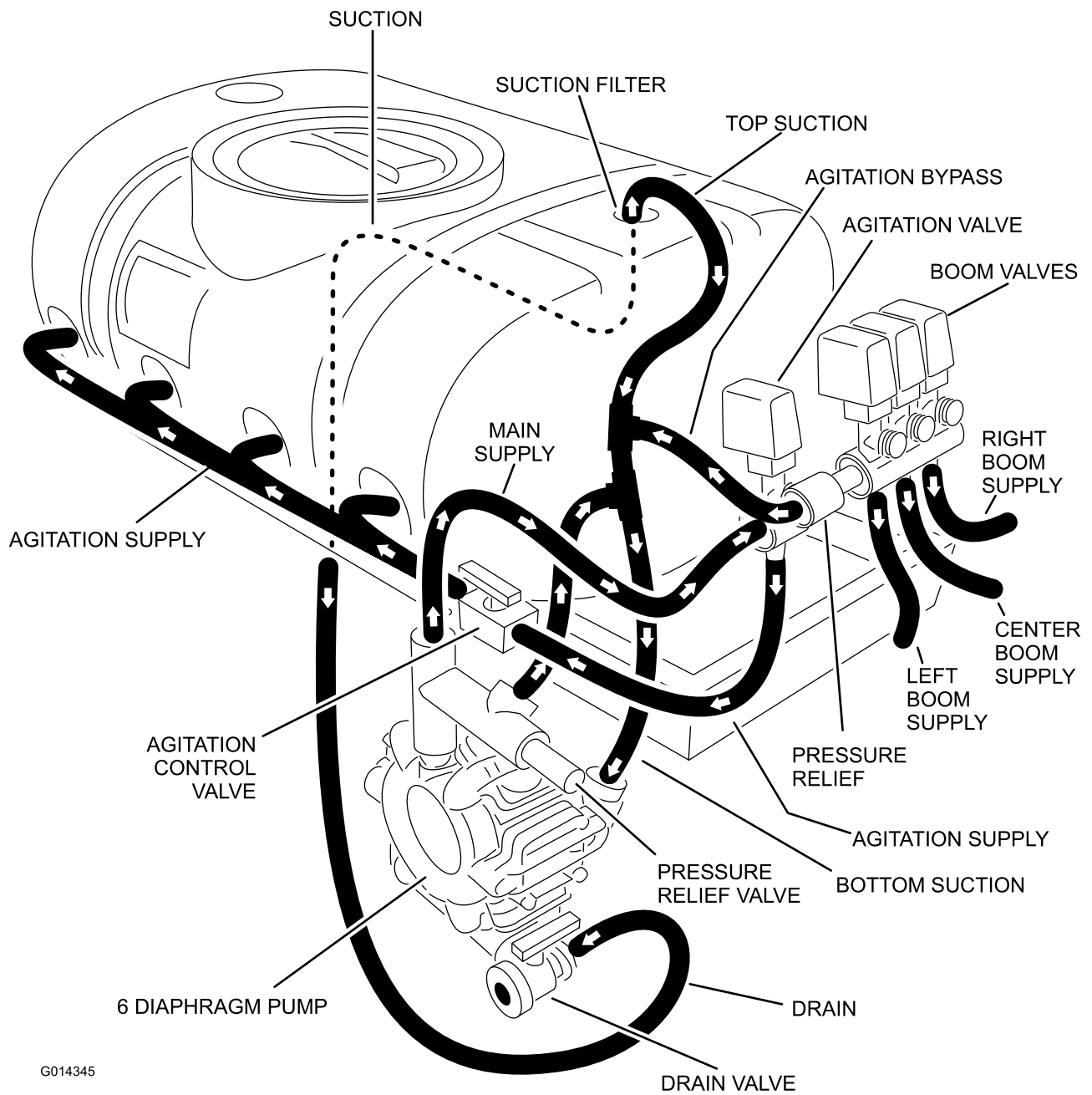
Schéma de principe (Rev. A)
