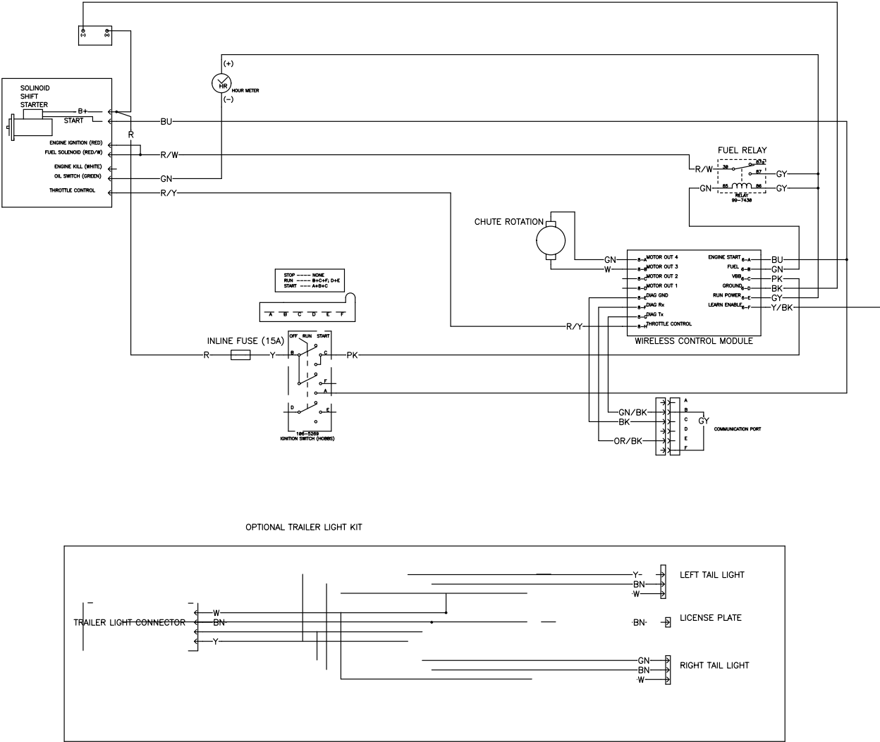
Kytkentäkaavio (Rev. -)
