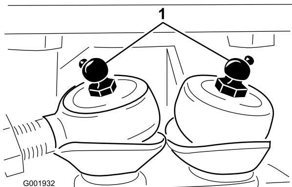
Figur 38 Styrstänger
