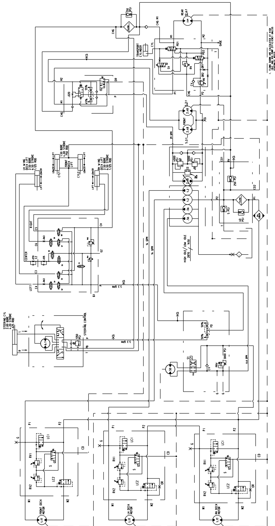
Hydraulisches Schema (Rev. B)
