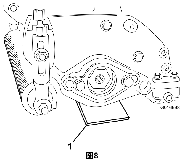
1. 调刀尺
