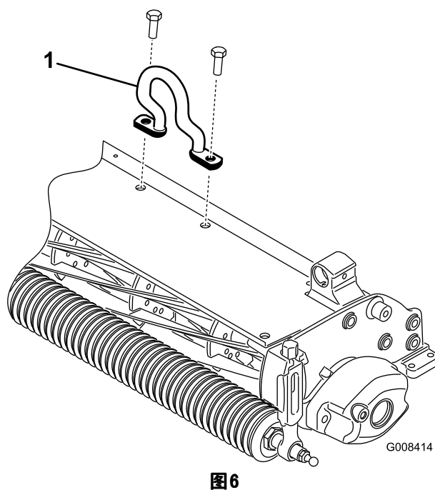
1. 偏置吊钩
