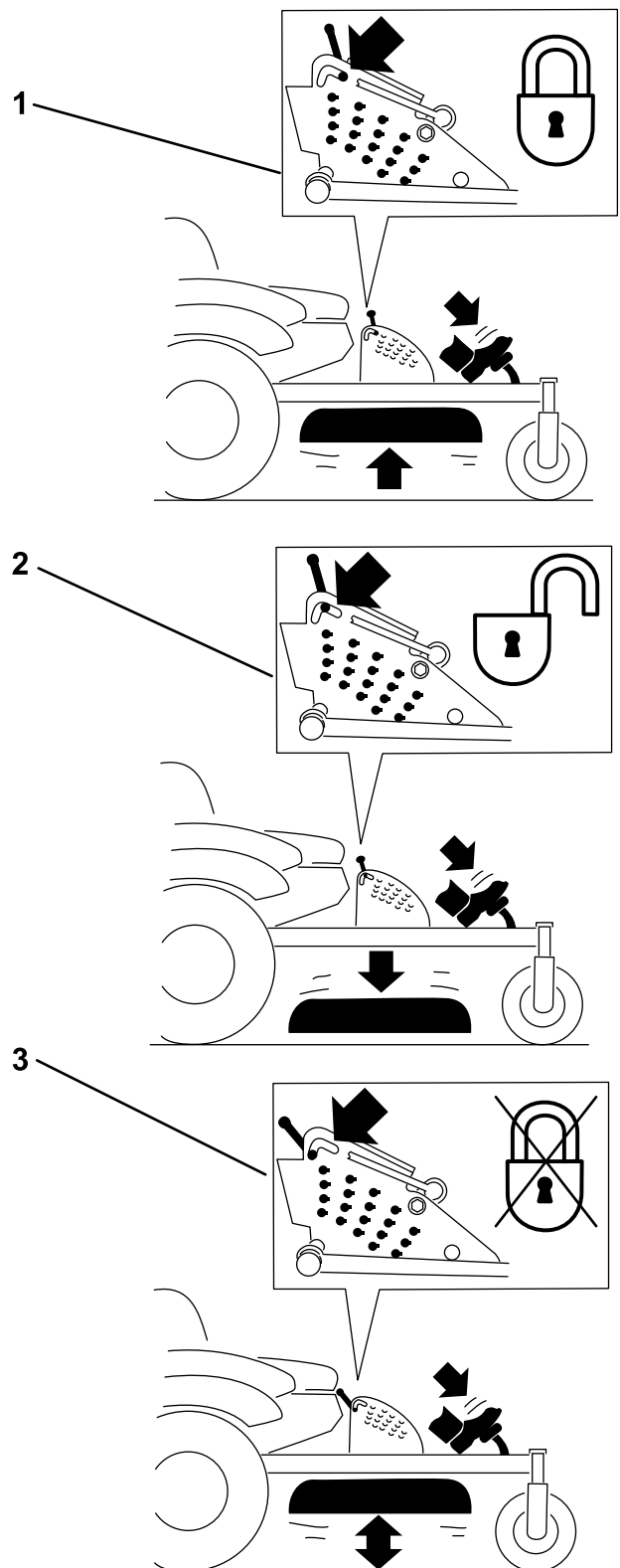
Bild 26 Transportriegel-Stellungen
