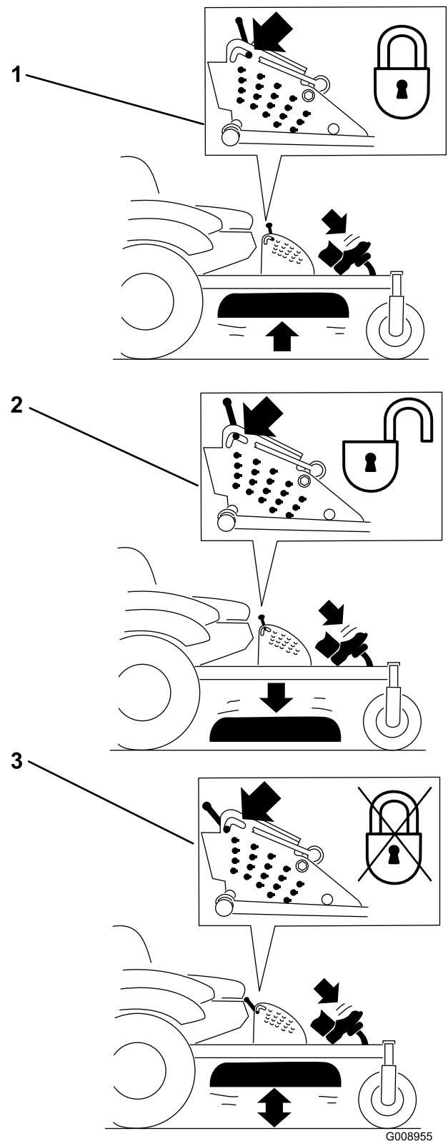
Figur 26 Transportlåspositioner
