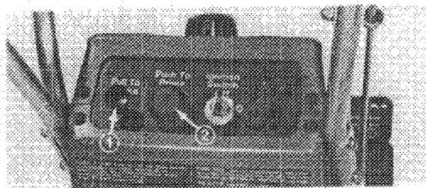
Figure 6 1. Choke 2. Primer
