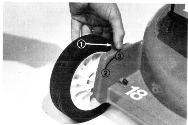
Figure 12 1. Dispositif de réglage de hauteur de tonte 2. Réglage haut 3. Réglage bas
