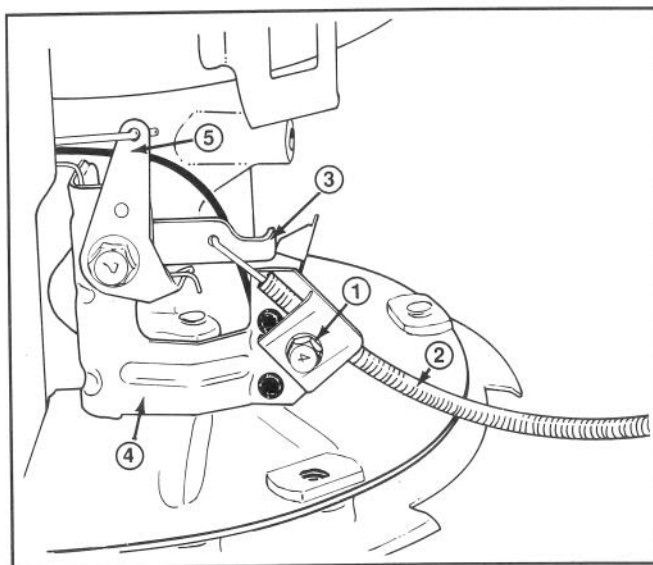
Posizione OFF (motore spento)
