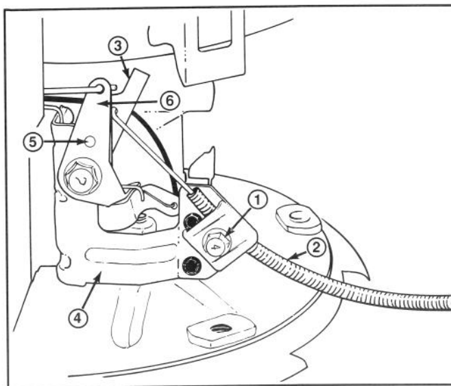
Posizione RAPIDO (velocità massima)
