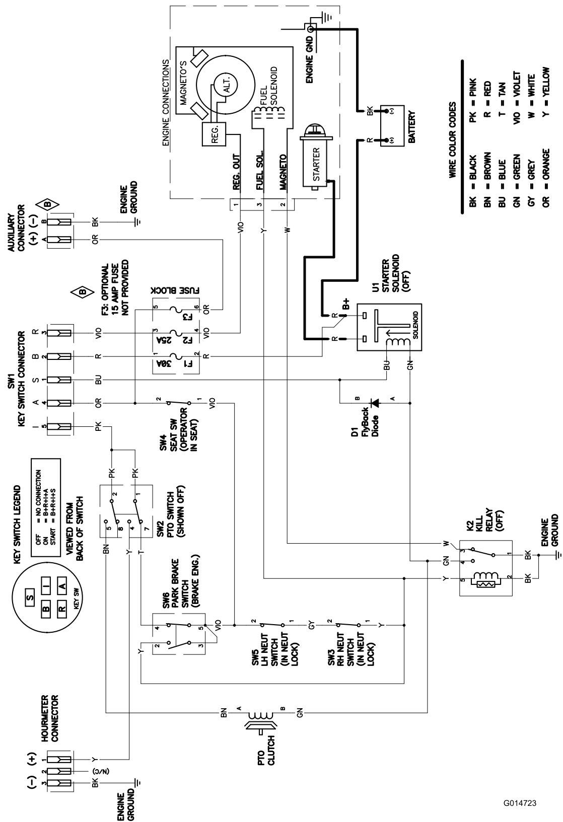
Diagrama de cabos (Rev. B)
