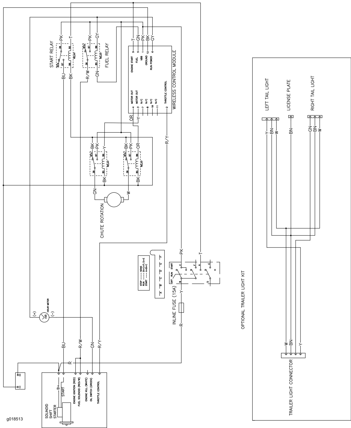
Elektronikkskjema (Rev. -)
