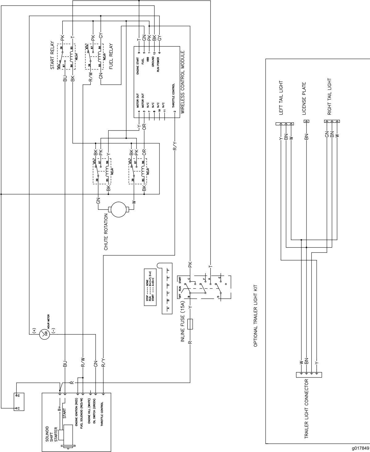
Elschema (Rev. -)
