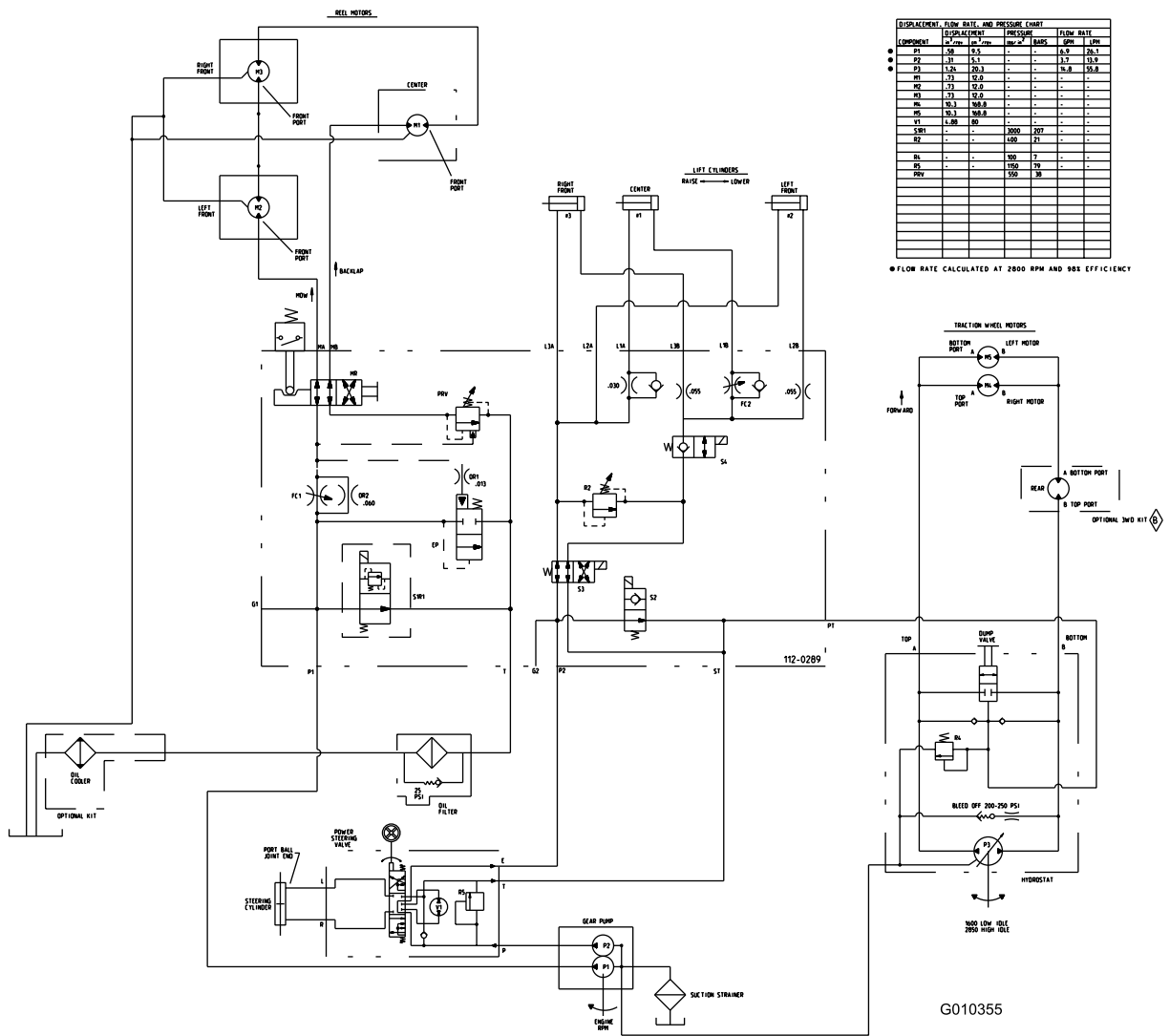
Hydraulikschaltplan (Rev. )
