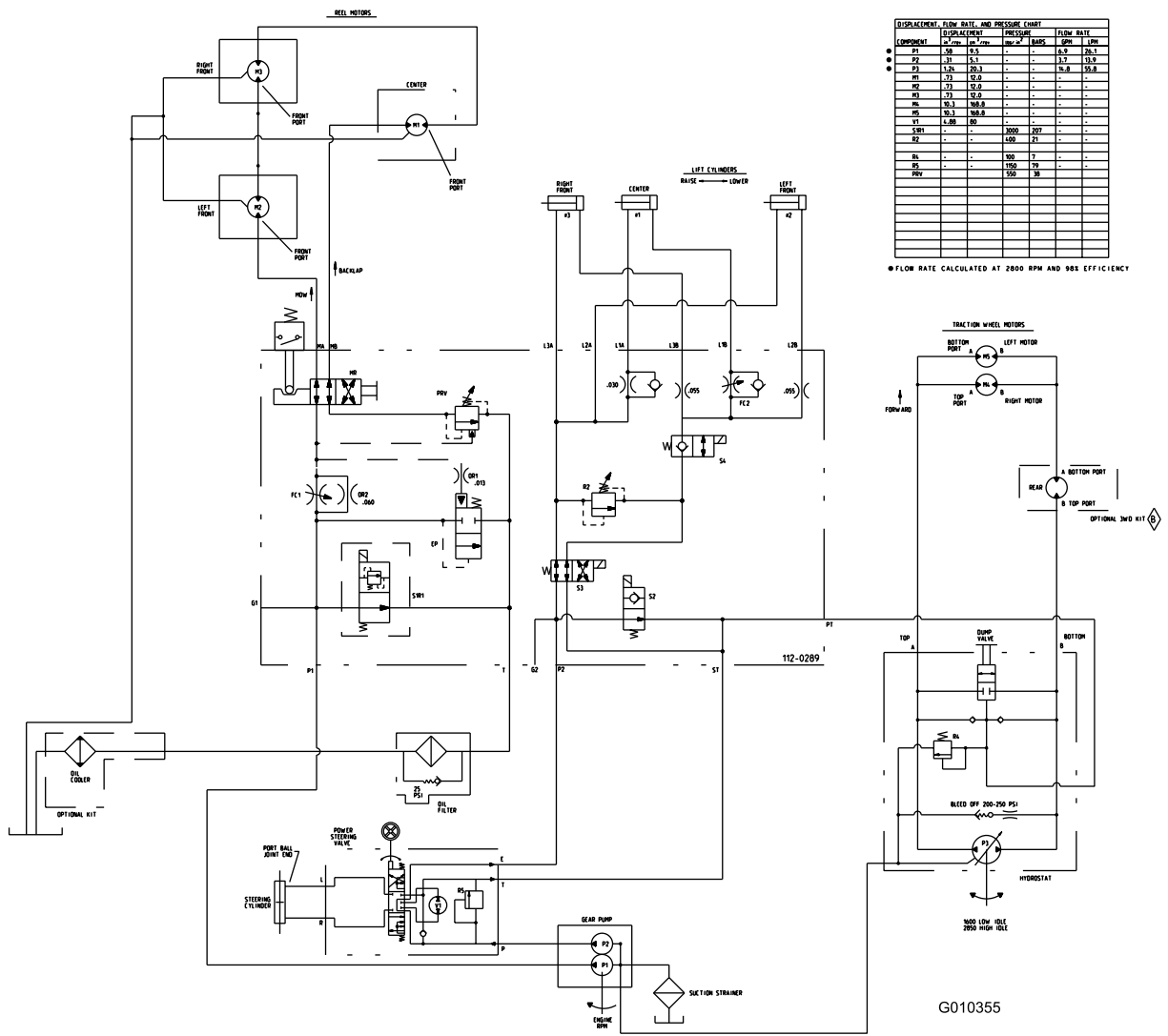
油压回路图 (Rev. )
