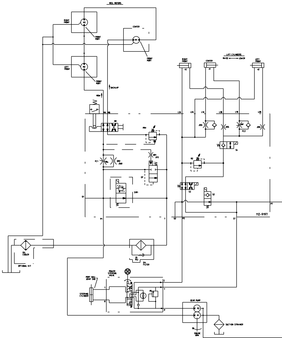
Schema idraulico (Rev. D)
