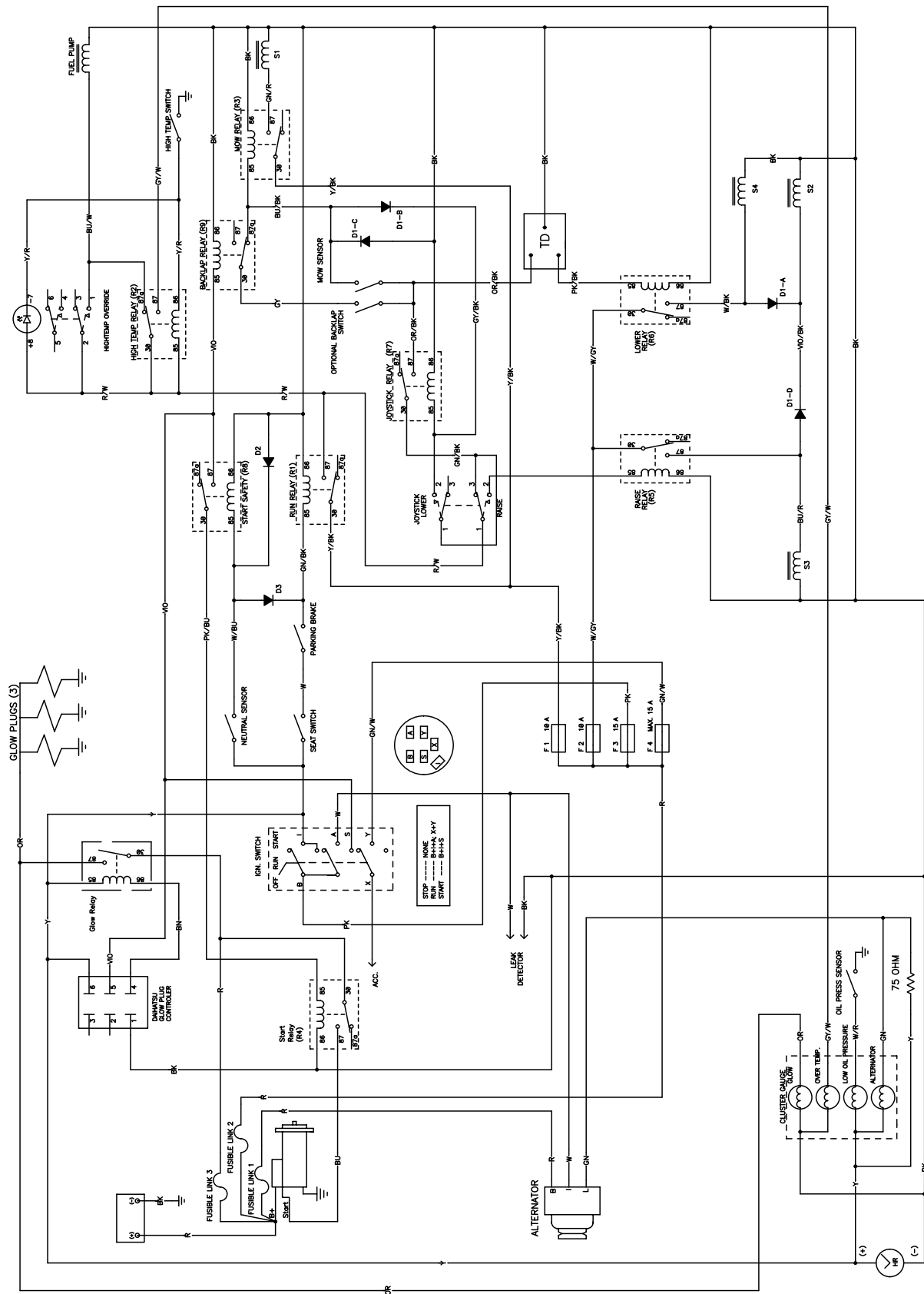
Elektronikkskjema (Rev. B)
