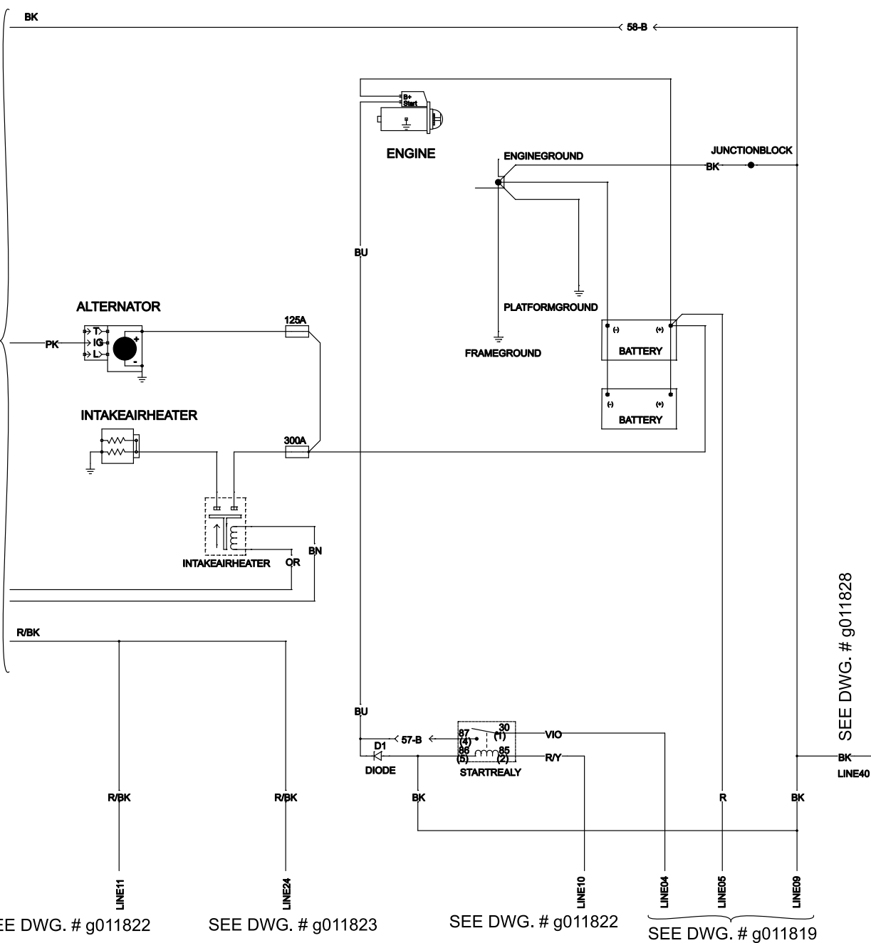
Esquema eléctrico (G011818) (Rev. A)
