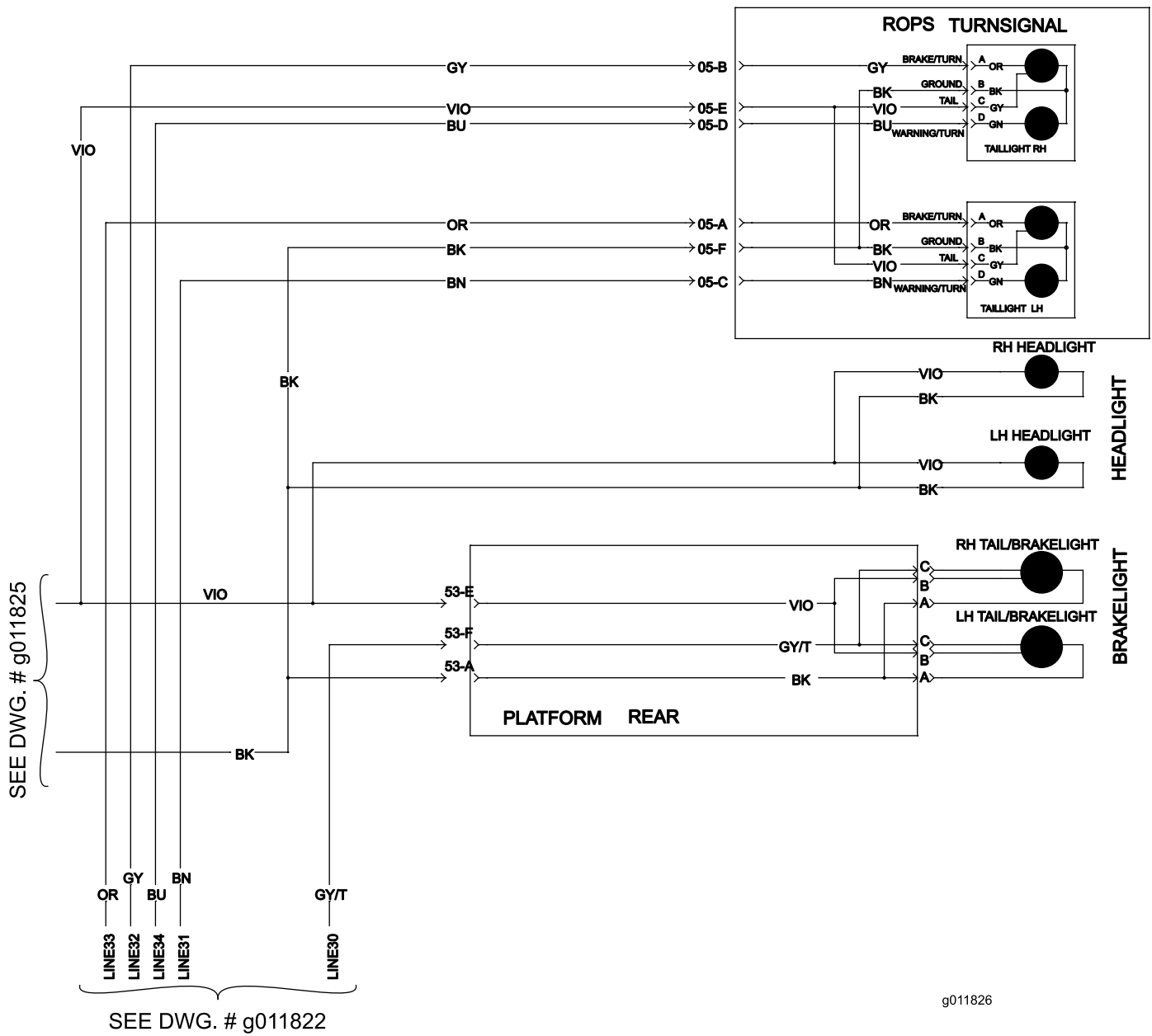
Esquema eléctrico (G011826) (Rev. A)
