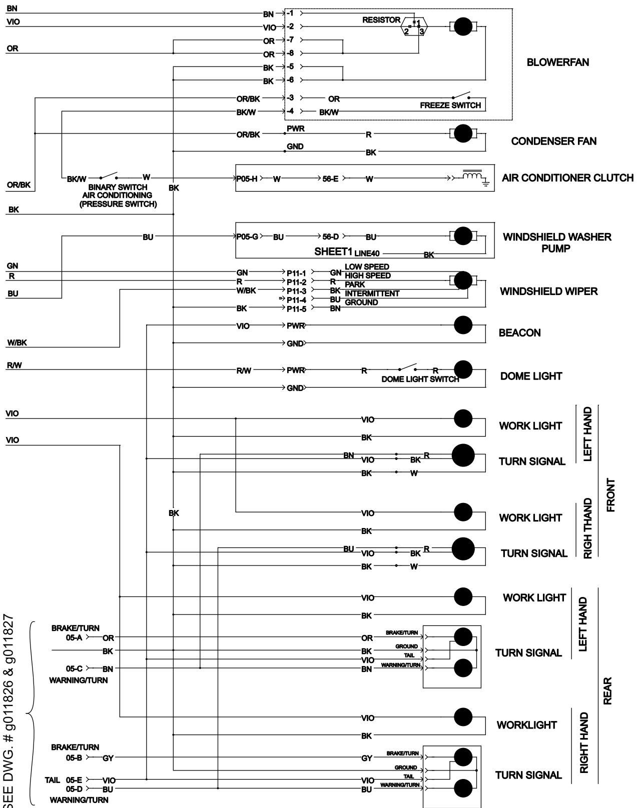
Kytentäkaavio (G011828) (Rev. A)
