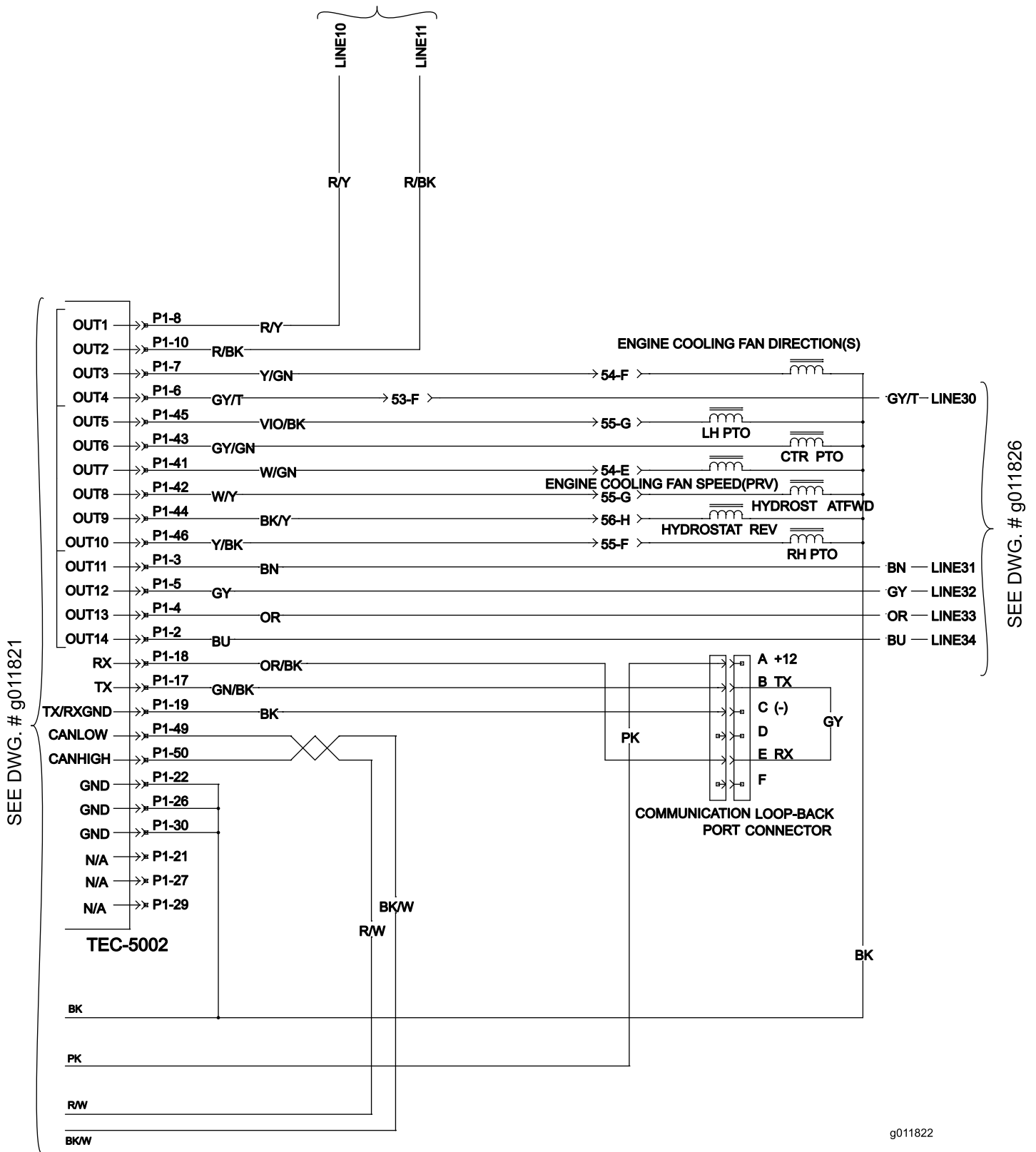
Kytentäkaavio (G011822) (Rev. A)
