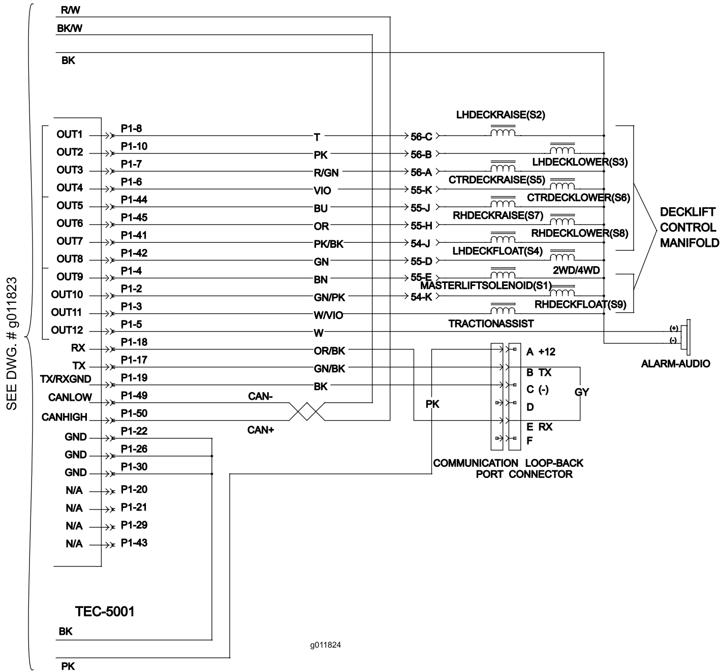
Kyt Kentäkaavio (G011824) (Rev. A)
