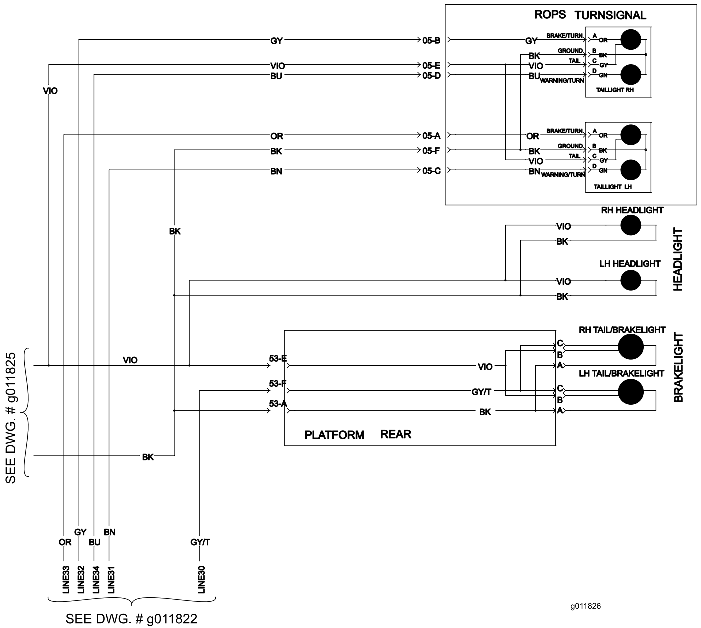
Kytentäkaavio (G011826) (Rev. A)
