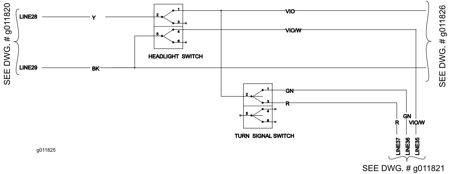
Kytcentäkaavio (G011825) (Rev. A)
