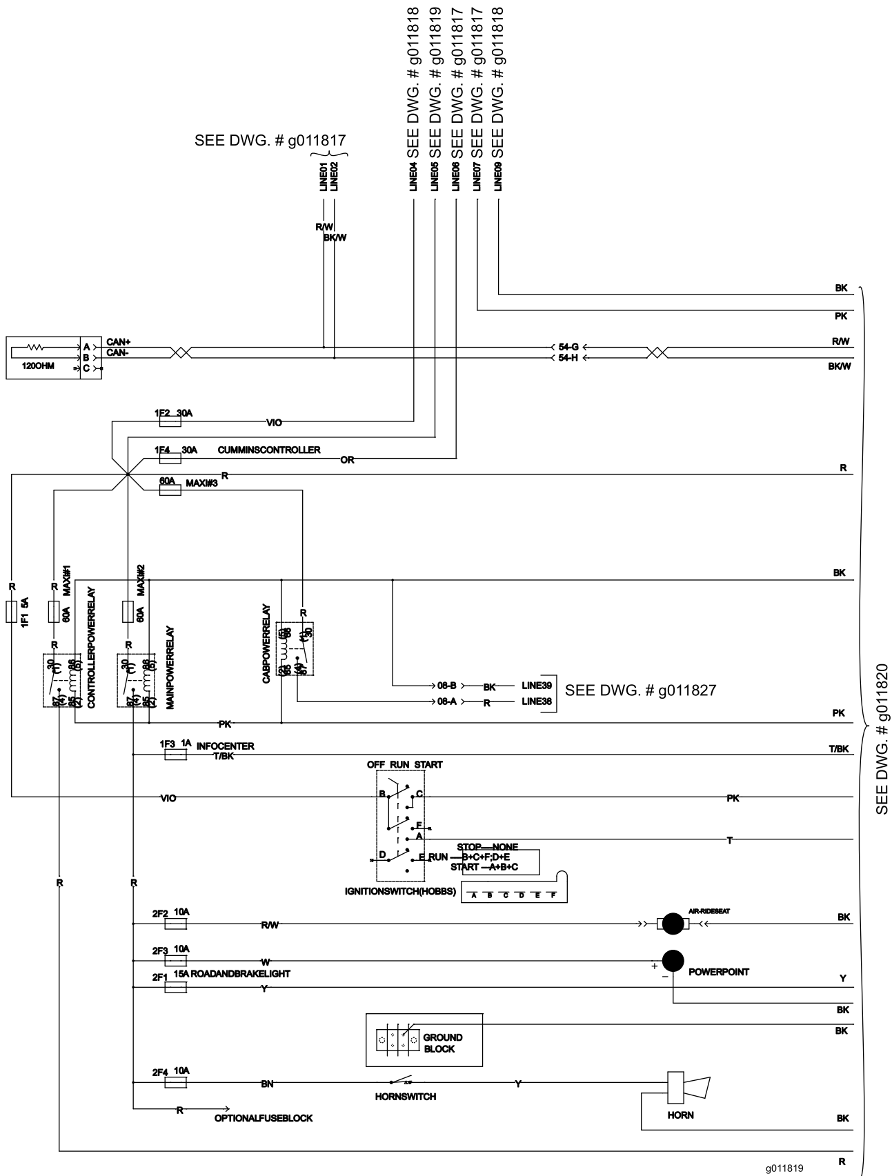
KytKentäkaavio (G011819) (Rev. A)
