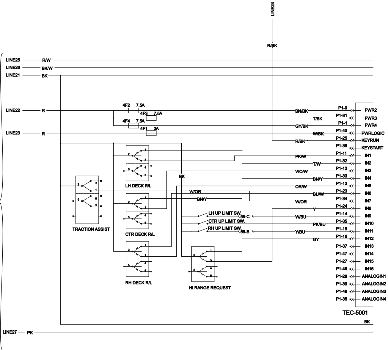
Kytcentäkaavio (G011823) (Rev. A)
