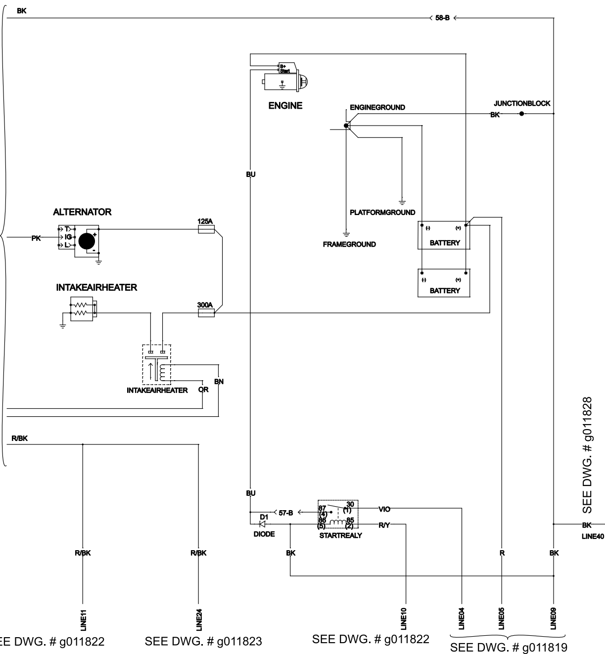
KytKentäkaavio (G011818) (Rev. A)
