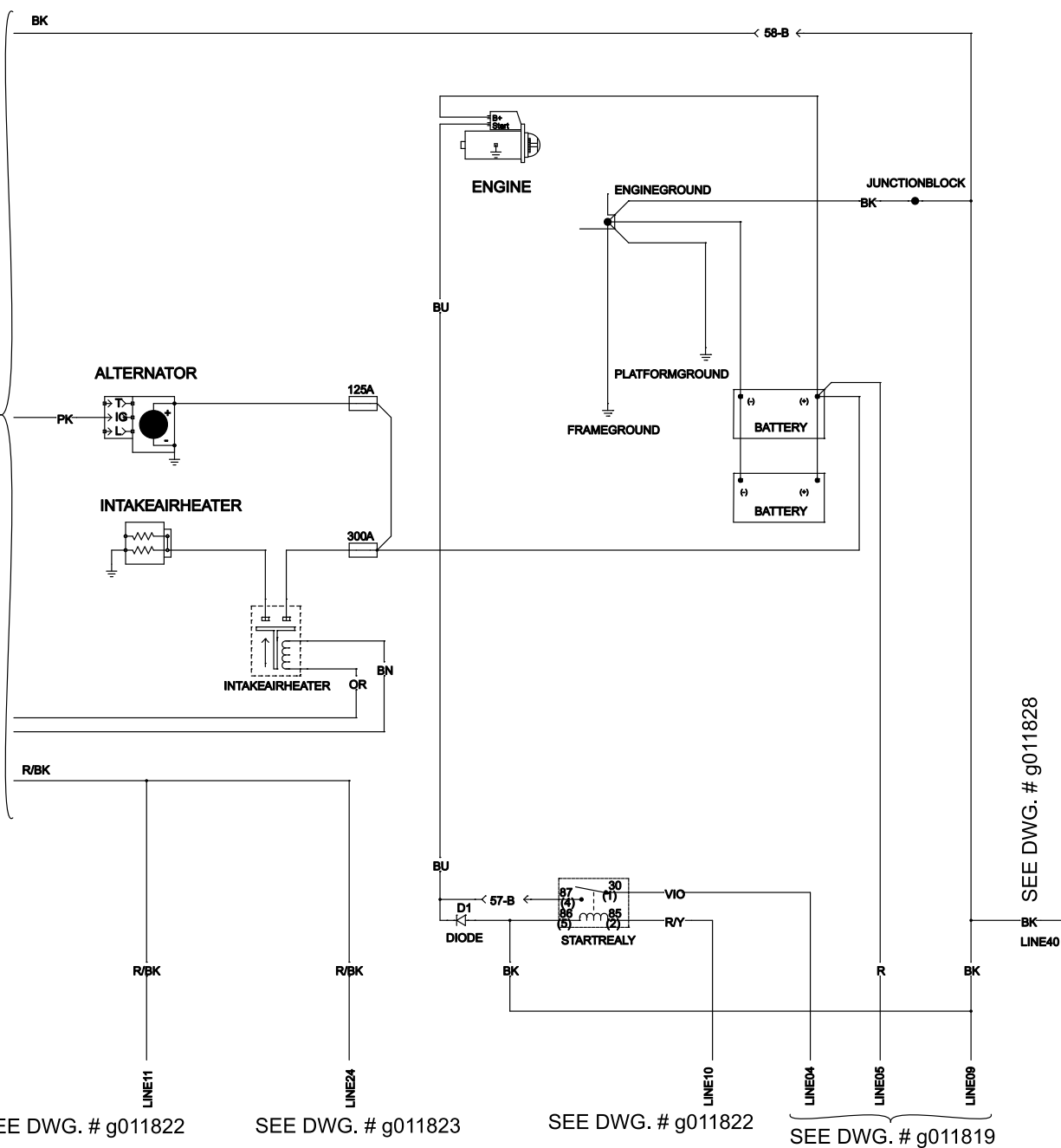
Schéma électrique (G011818) (Rev. A)
