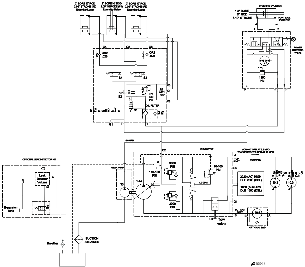
Schéma hydraulique (Rev. A)
