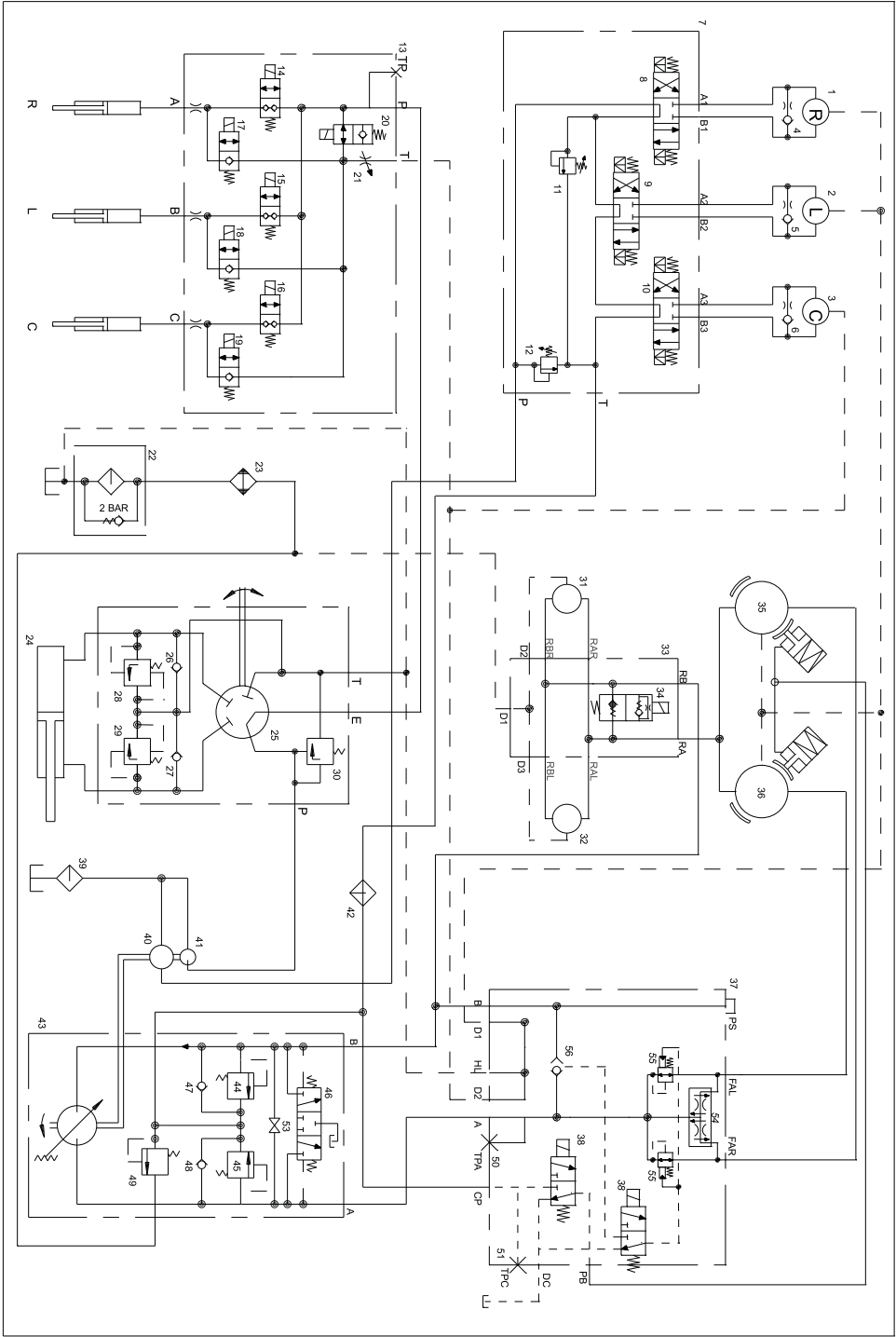
Ledningsdiagram, LT 3340 (Rev. A)
