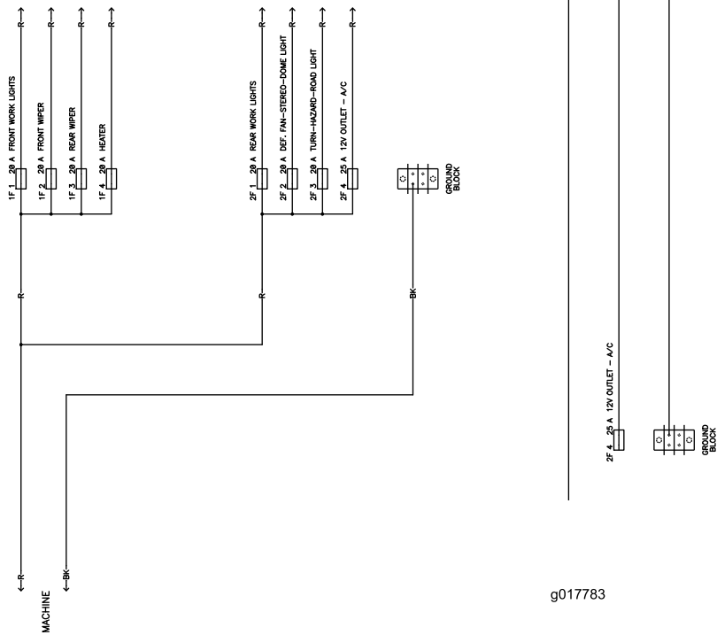
Schéma électrique - GM 4110 (Rev. D)
