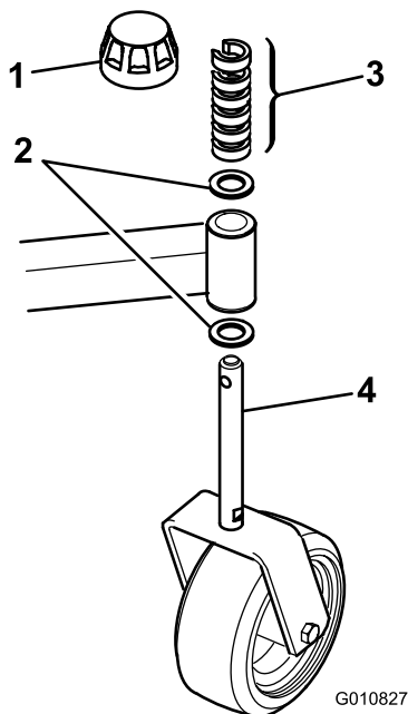
Figur 3 Bakre styrehjulsenhet
