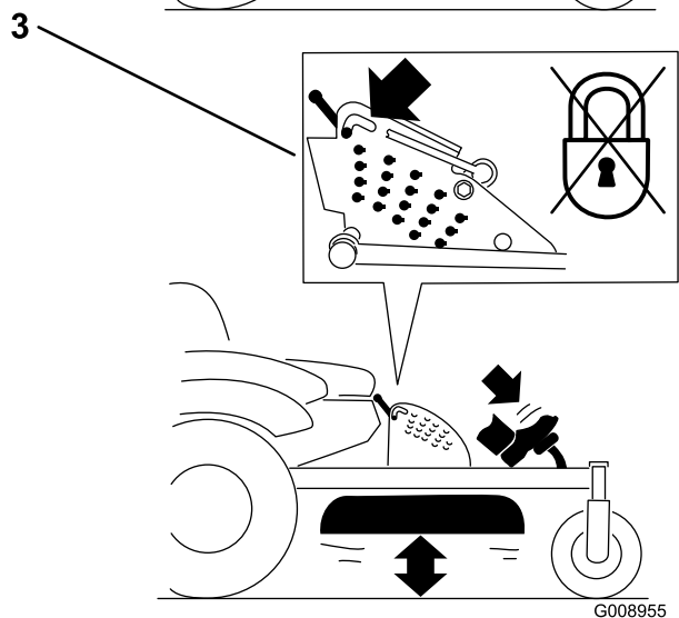
Figur 26 Transportlåsstillinger
