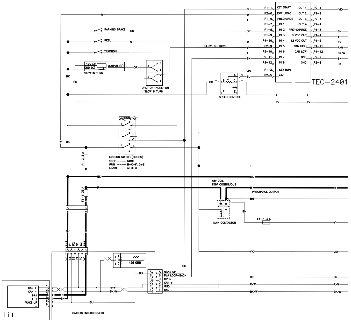
Esquema eléctrico, Parte 1 (Rev. A)
