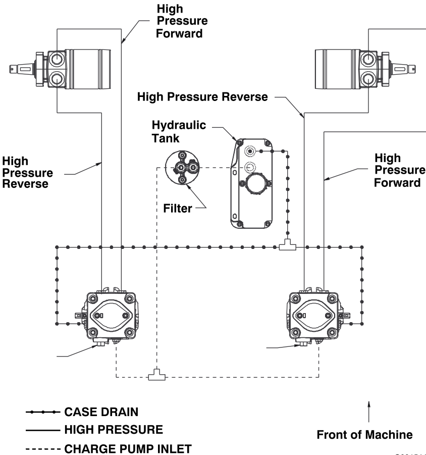
Esquema hidráulico (Rev. A)
