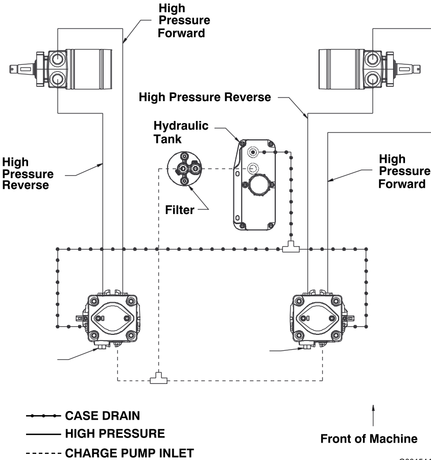
Schéma hydraulique (Rev. A)
