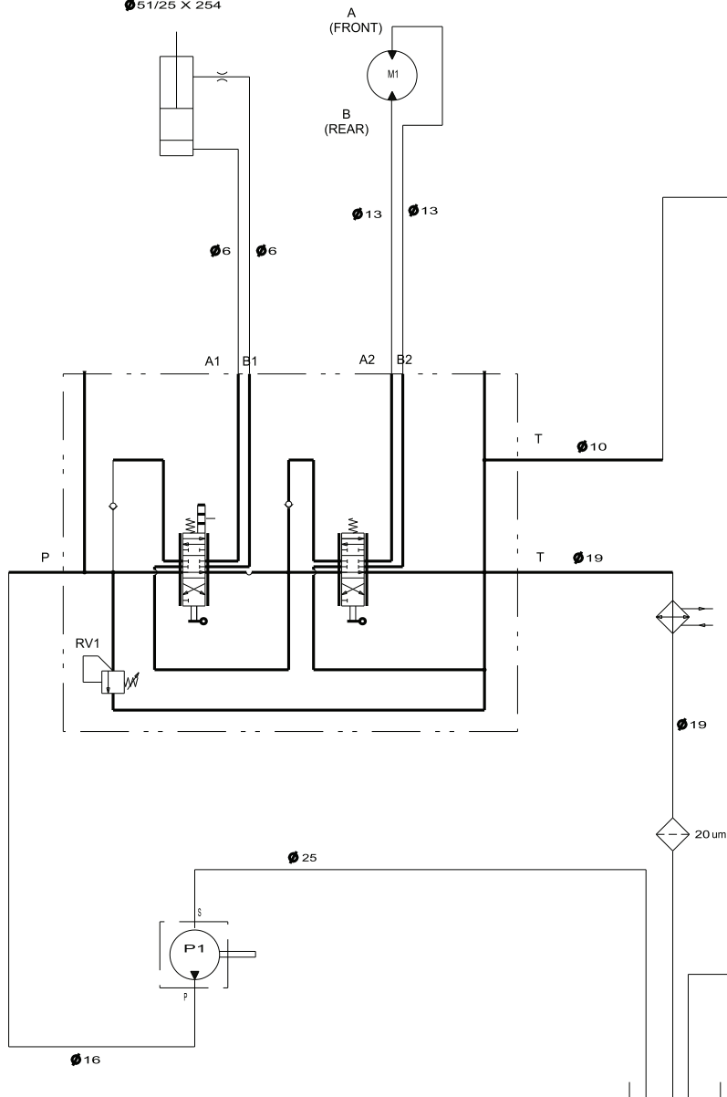
Hydraulschema (Rev. B)
