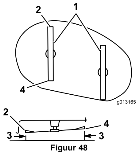
Figuur 48 Boven- en zijaanzicht van maaibehuizing
