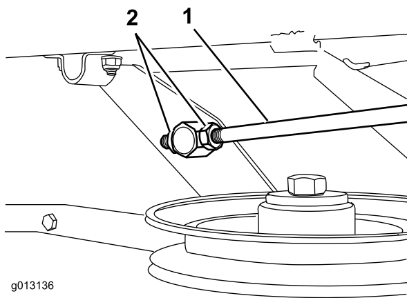
Figuur 44 Linkerzijaanzicht
