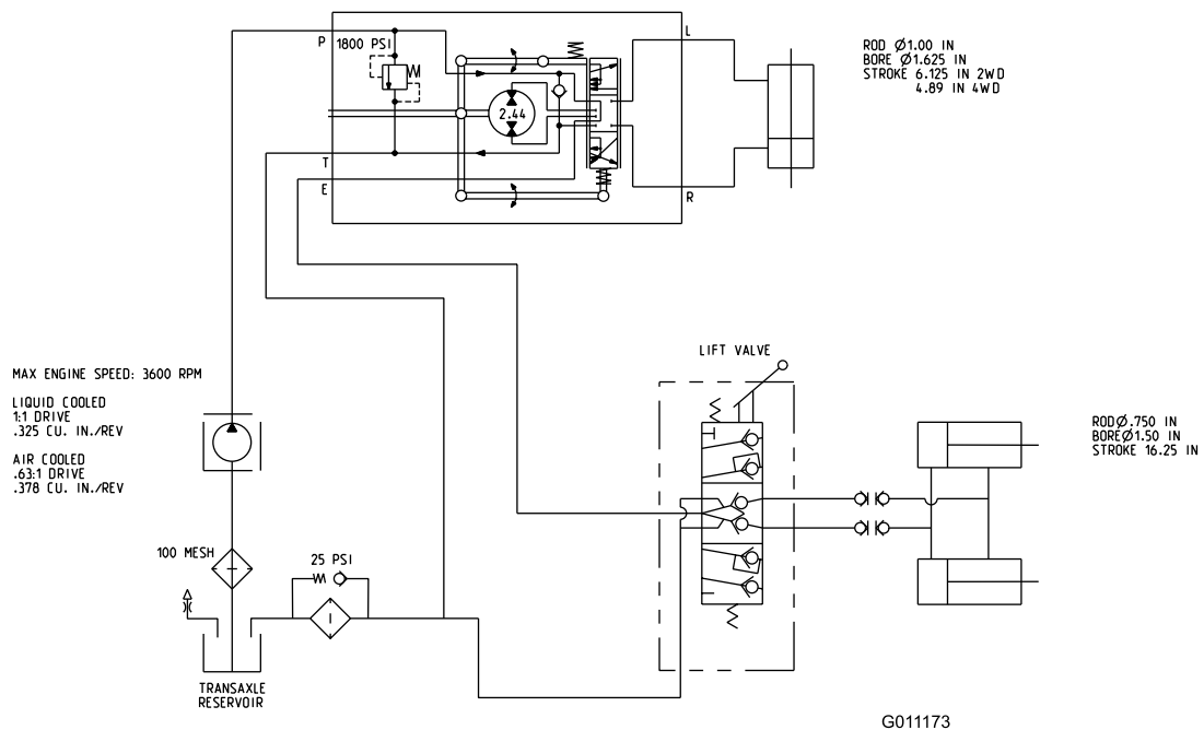
Schéma hydraulique (Rev. B)
