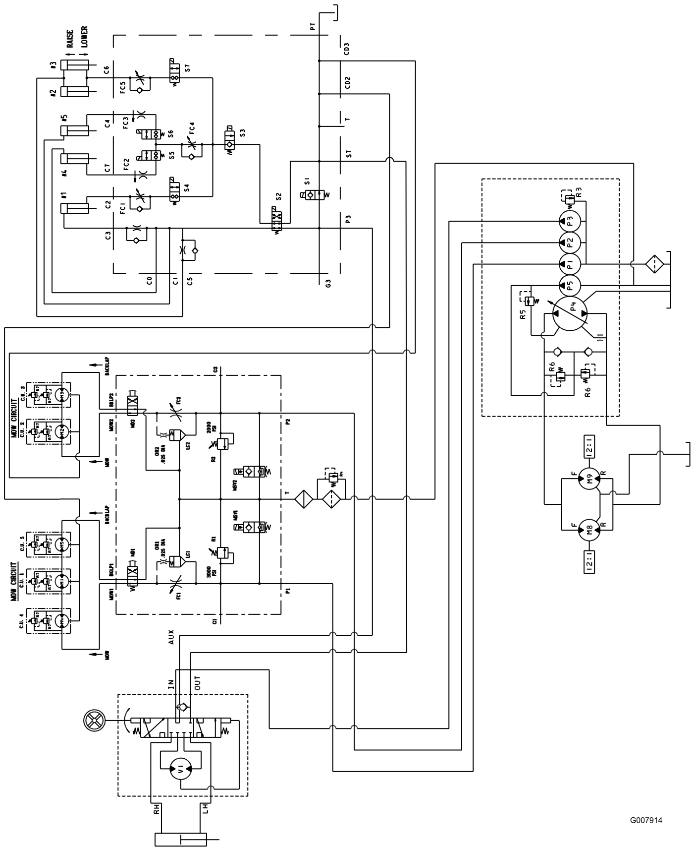
Hydraulikschemata, Modell 03806 (Rev. -)
