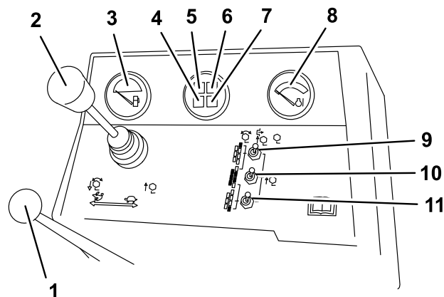
Figura 22 Modelos 03808 e 03813
