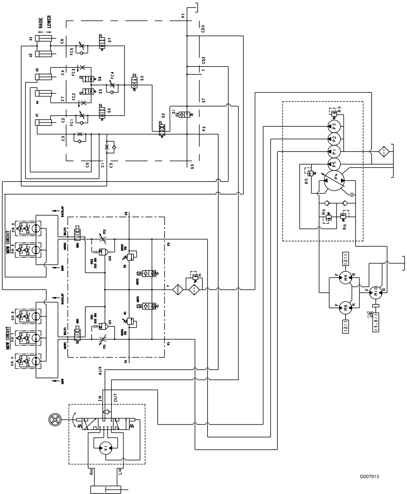
Hydraulschema, modellerna 03807 och 03812 (Rev. -)
