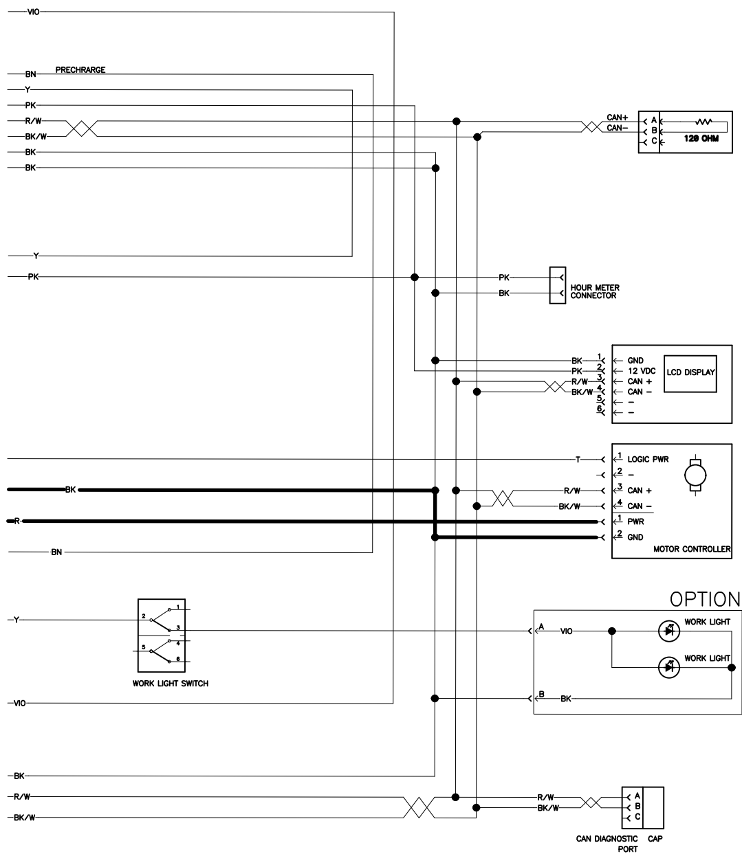
Elektrické schéma, část 2 (Rev. A)
