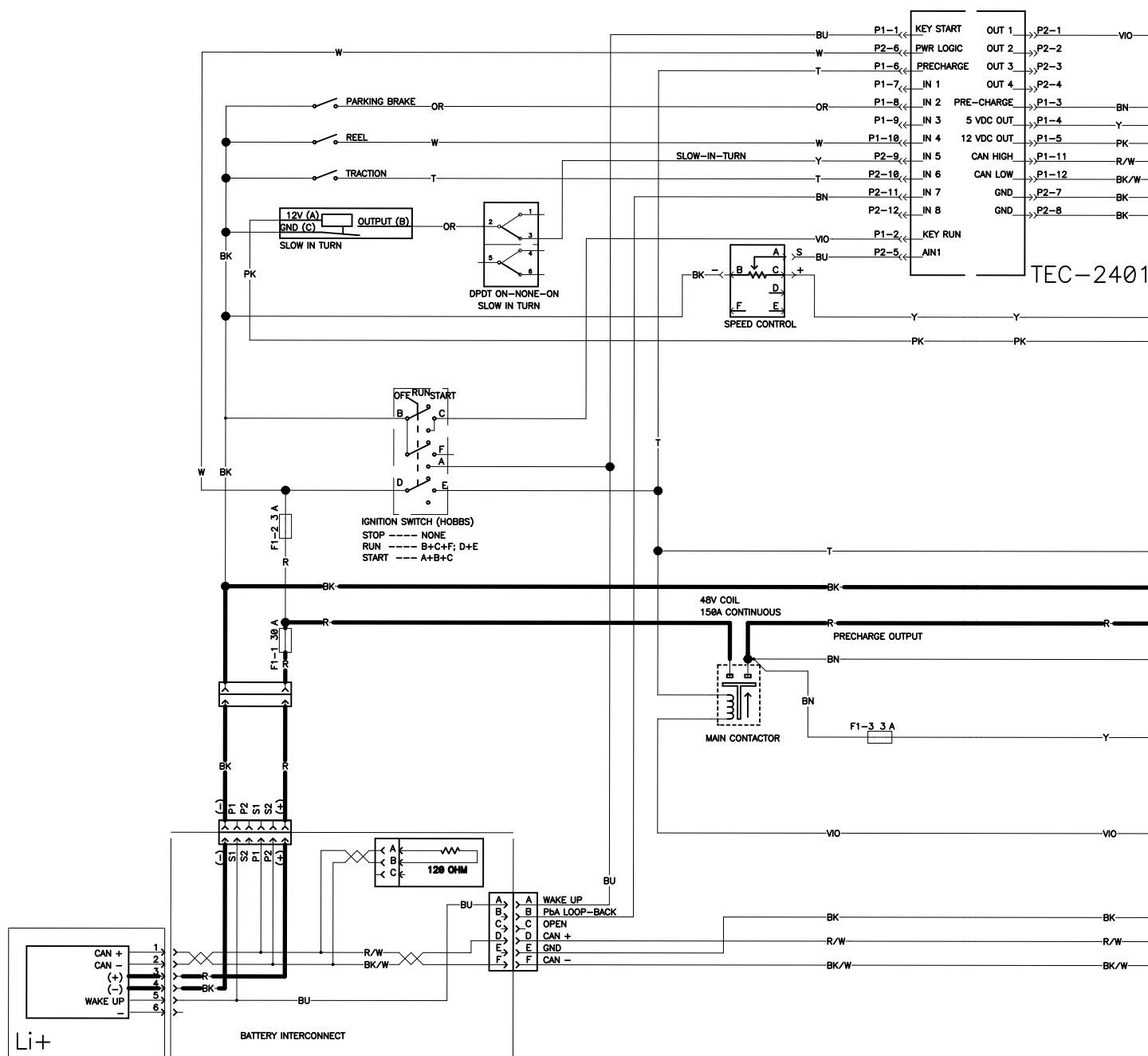
Elektrické schéma, část 1 (Rev. A)
