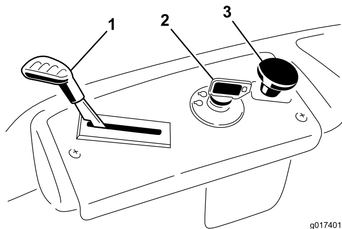
Figuur 5 Bedieningspaneel
