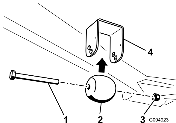
Kuva 12 Vain Guardian-leikkurit
