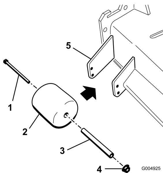
Kuva 13 Vain sivuheittoleikkurit
