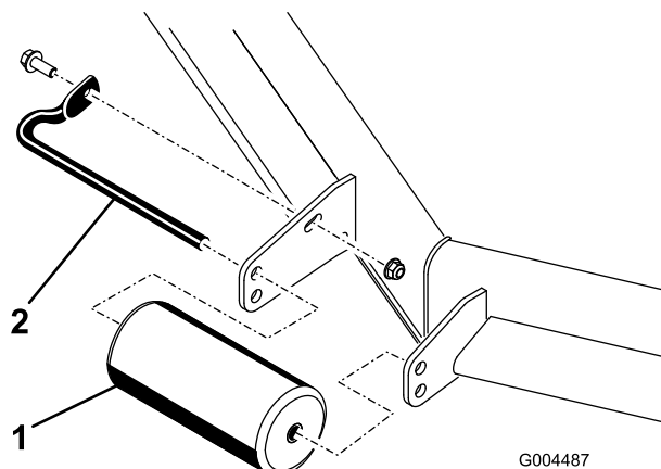
Figur 10 Alla gräsklippare
