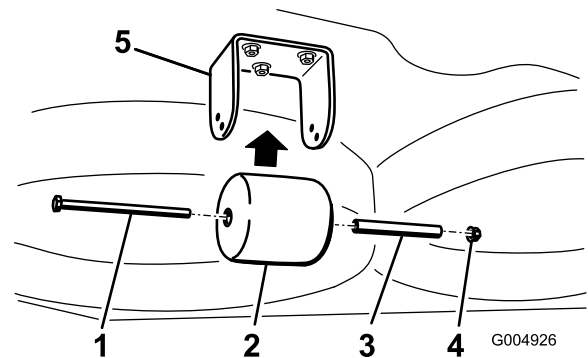
Figura 21 Solo piatti di taglio del tosaerba Guardian
