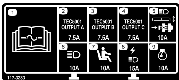
Modelos de tracção às 4 rodas
