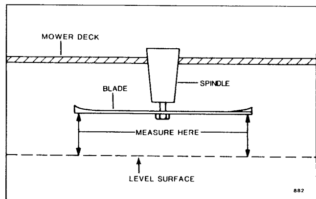
FIG. 7 Blade Level
