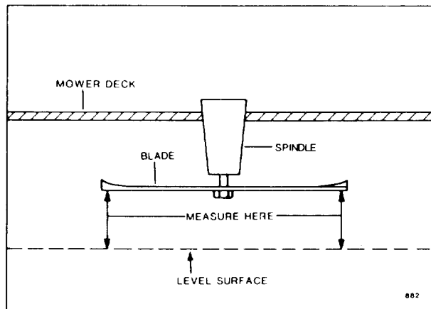
FIG. 6 Blade Level
