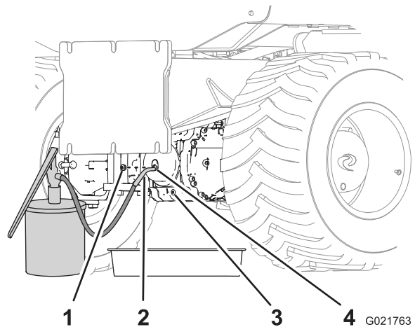
Bild 69 Hinterachse
