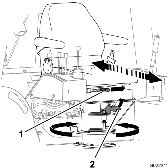
1. Schaltbügel
