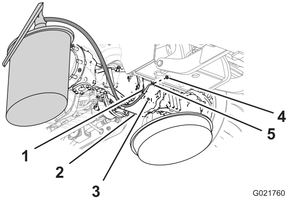
Figura 68 Eixo dianteiro
