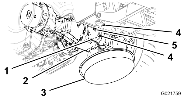
Figura 66 Eixo dianteiro
