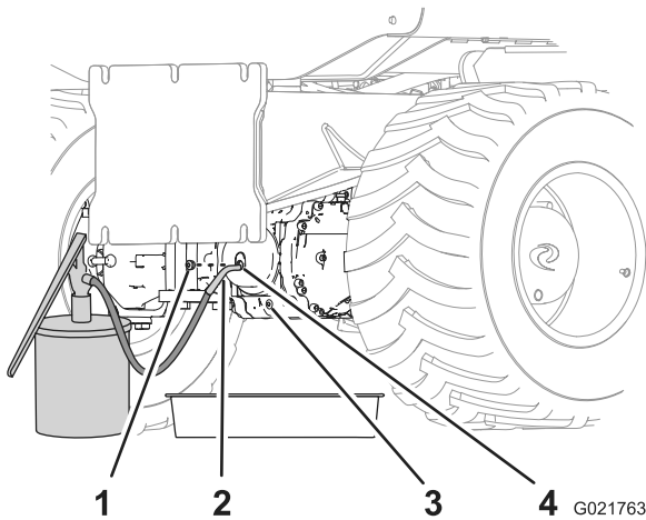
Figura 69 Eixo traseiro
