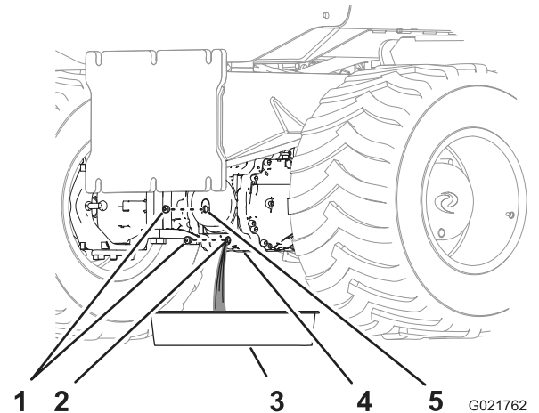
Figura 67 Eixo traseiro
