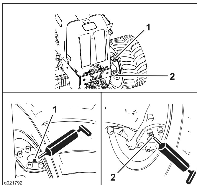
Figura 30 Eixo dianteiro
