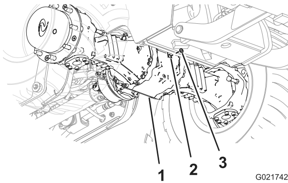
Figura 64 Eixo dianteiro
