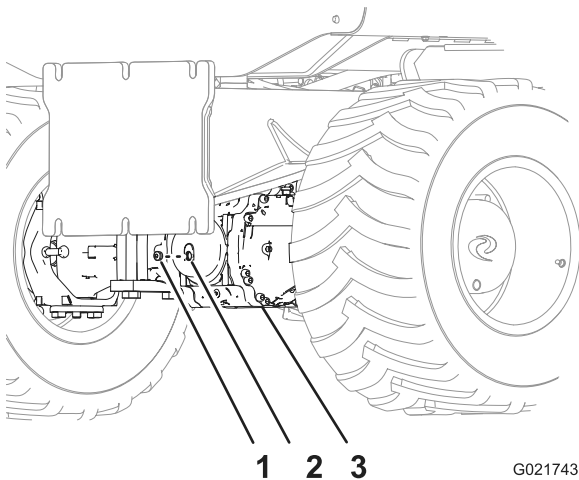
Figura 65 Eixo traseiro
